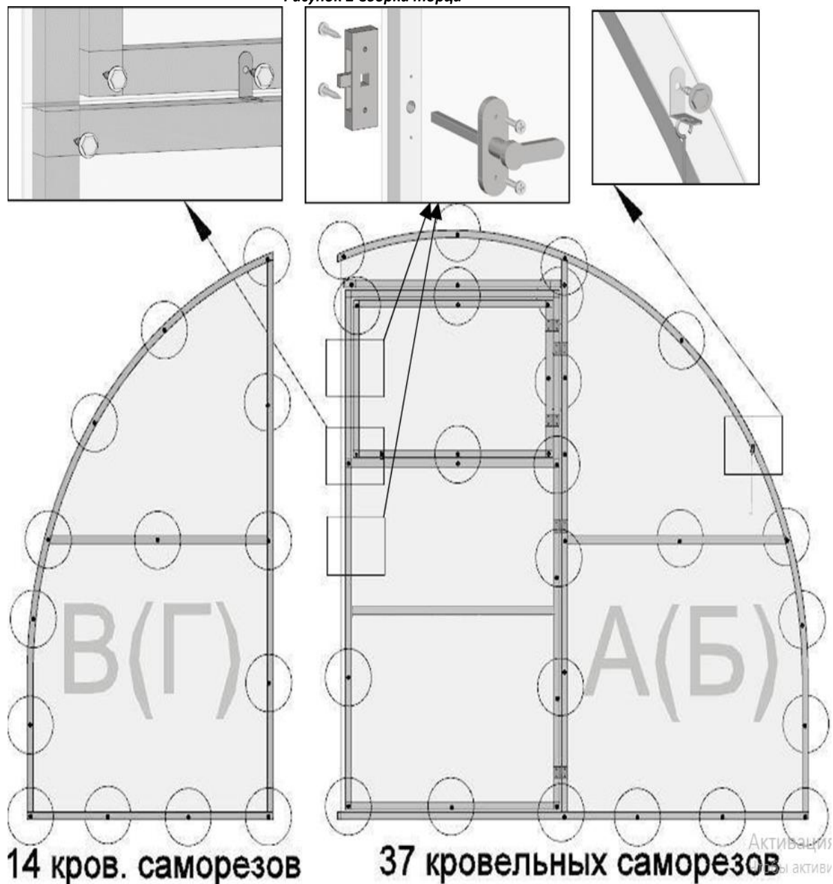
Рисунок 2 Сборка торца
