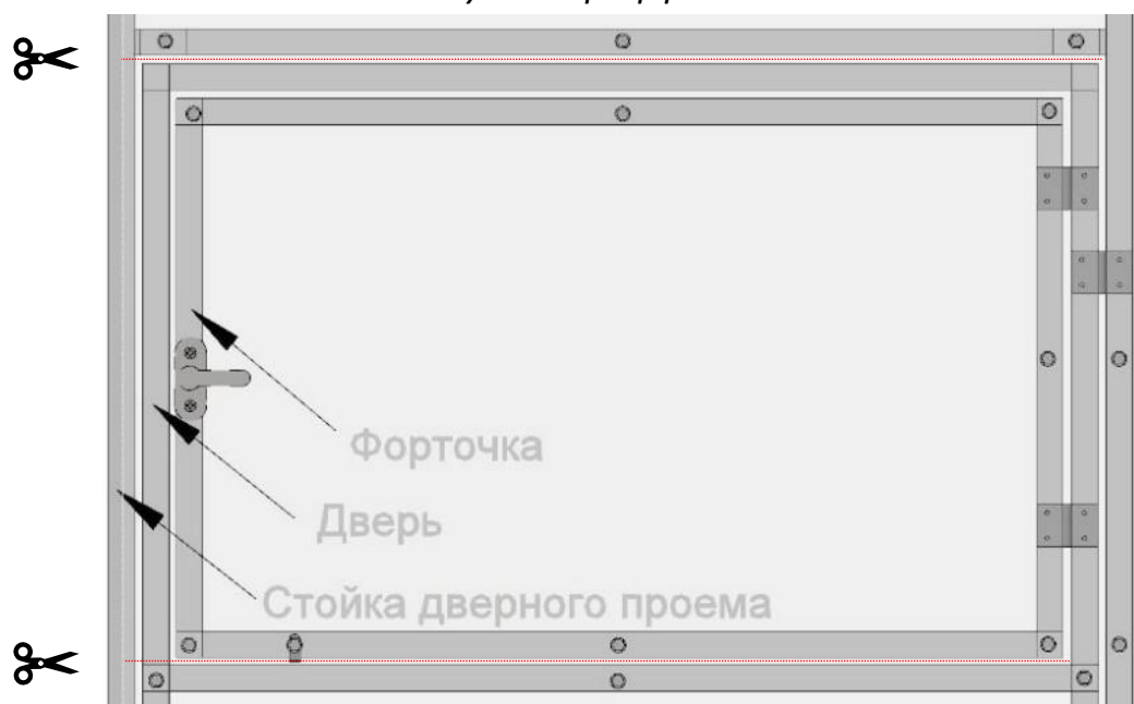
Рисунок 3 Сборка форточки
