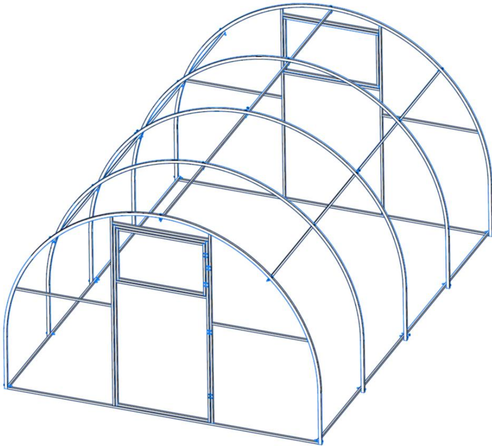
Схема компоновки «Удлинение +2м»
