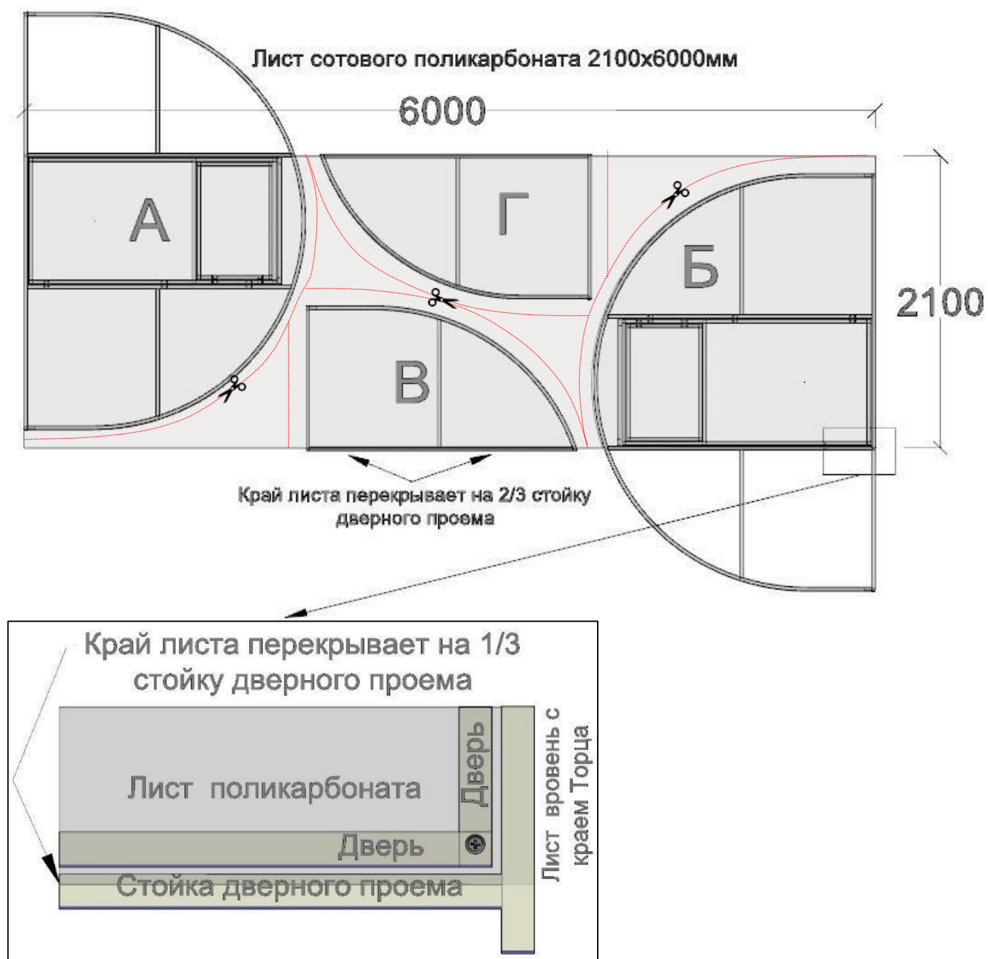
Рисунок 1 Лист поликарбонат раскрой
