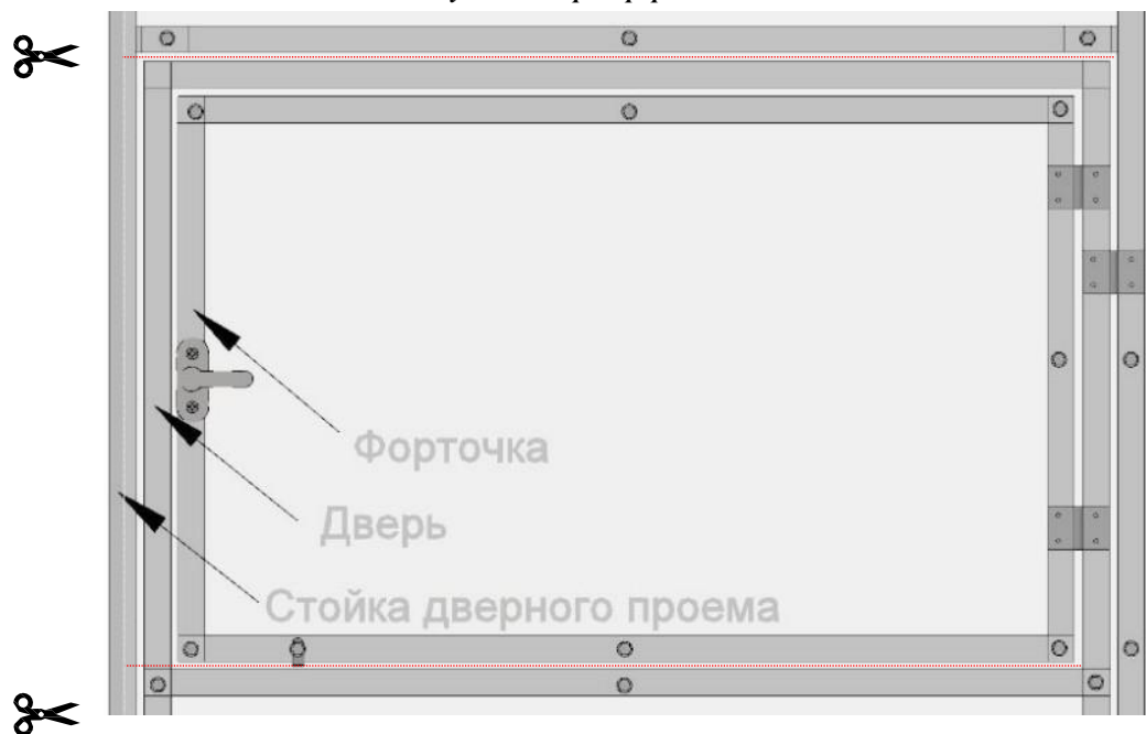
Рисунок 3 Сборка форточки
